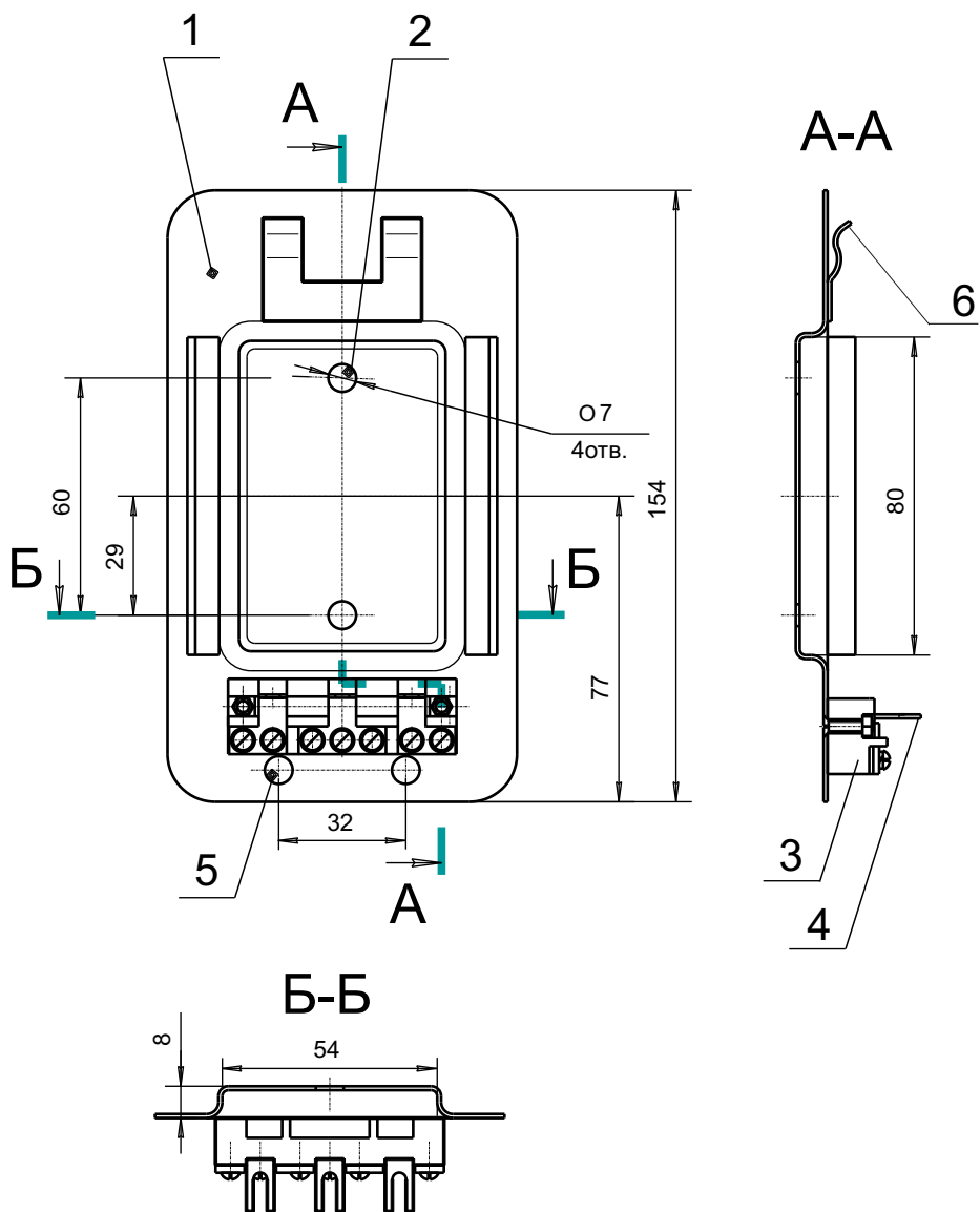
Рис. 2. Основание извещателя “Пульсар 3-01”
